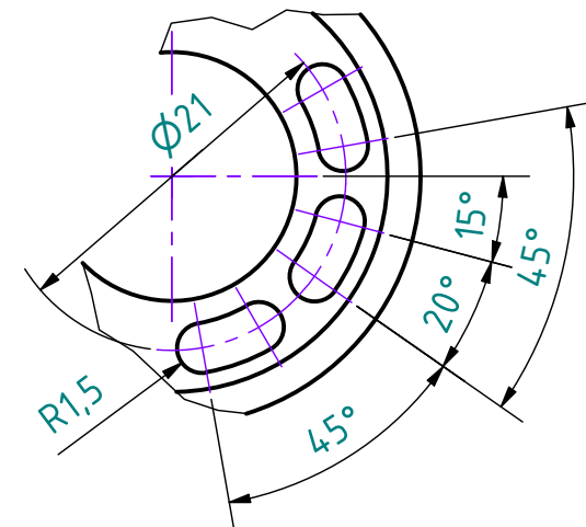
Detail D 2 : 1
